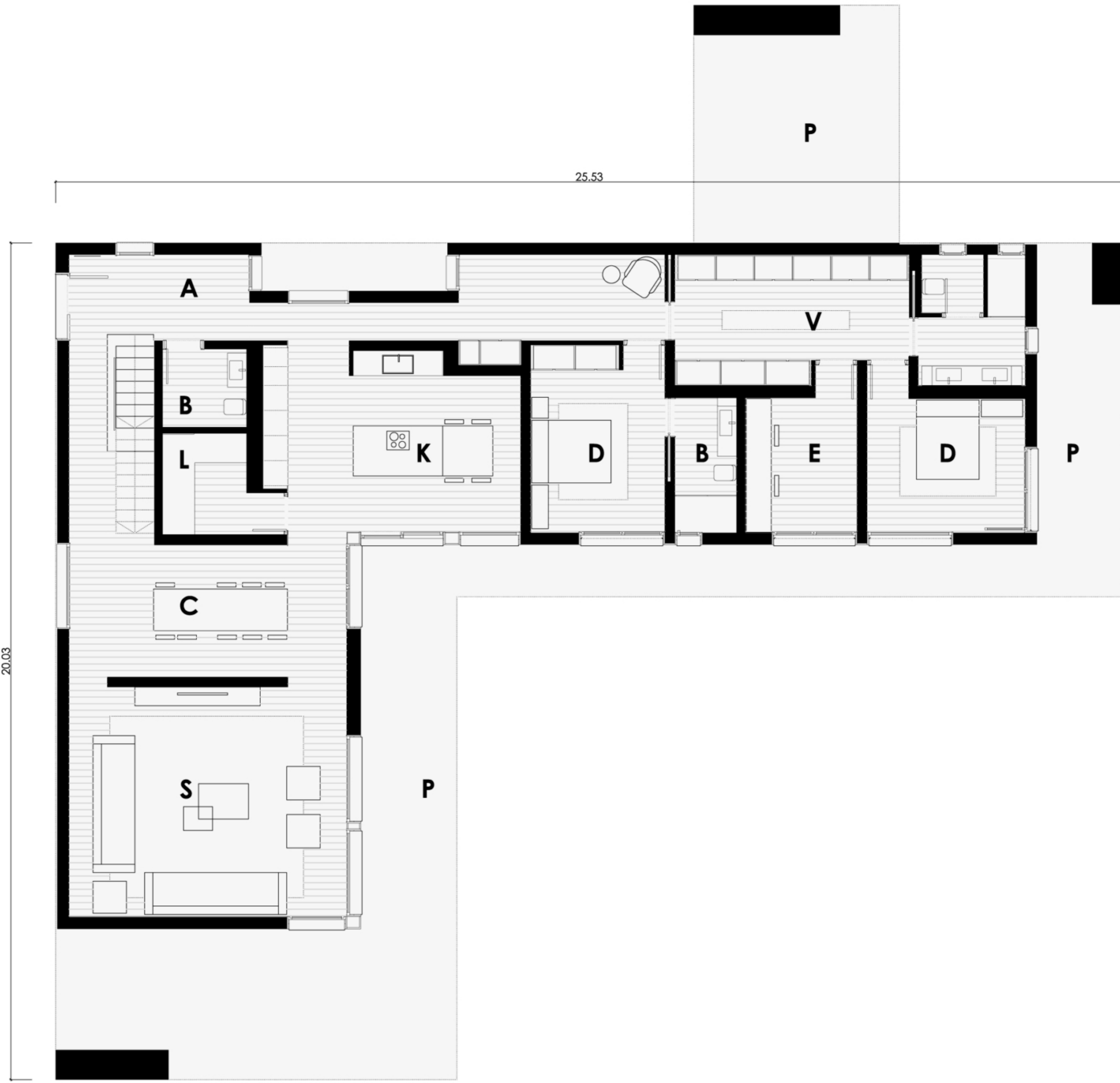
0 0.5 1 m PLANTA BAJA
